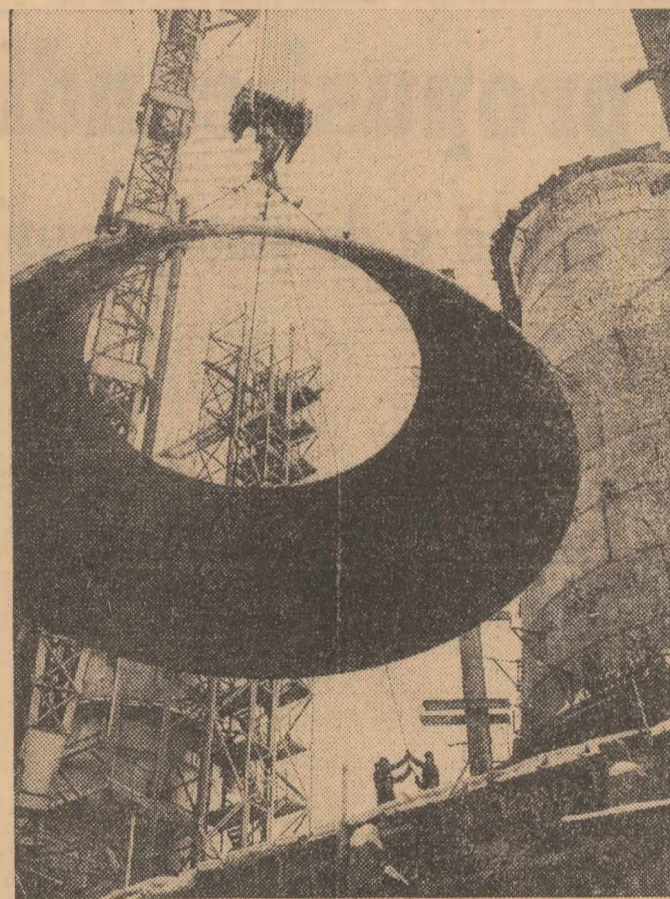
Moment de seamă pe șantierul celui de-al doilea furnal de 1700 mc al Combinatului siderurgic Galați. Brigada complexă condusă de încercatul montor Nicolae Foltozan, ridică cupola furnalului, ultimul ansamblu pe verticala corpului masivului agregat
