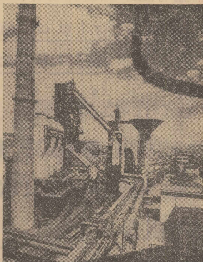
La Combinatul siderurgic din Hunedoara vor intra anul viitor în producție două cuptoare electrice de 50 tone cu o capacitate anuală de circa 120.000 tone oțeluri aliate. În clădire: unul din furnalele de 1.000 mc din cadrul combinatului. Foto: AGERPRES
