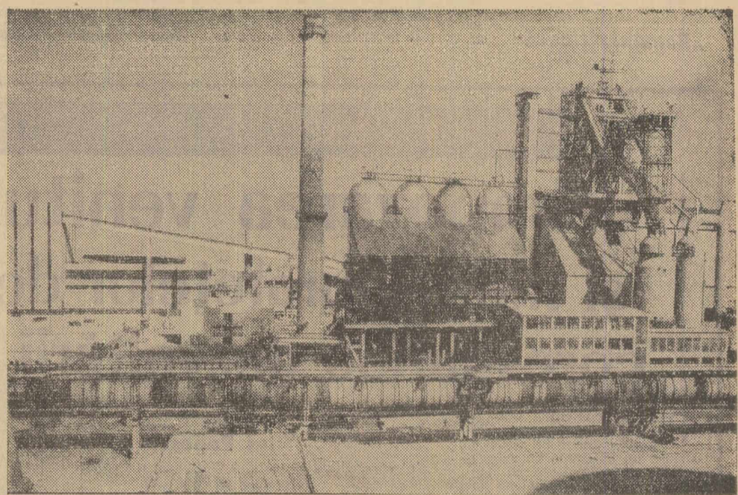
Furnalul de 1700 mc, care funcționează de peste șase luni la Combinatul siderurgic din Galați, este cel mai mare din țară și primul dintr-o baterie de patru care se vor construi aici. El produce două tone de fontă la fiecare minut, iar când va atinge în întregime parametrii va produce de șase ori cantitatea de fontă elaborată în 1948 în întreaga țară. Când vor fi date în folosință cele patru agregate gălățene vor realiza o producție anuală de 33 de ori mai mare decât a României antebelice. În clișeu: O vedere de ansamblu la furnalul 1
