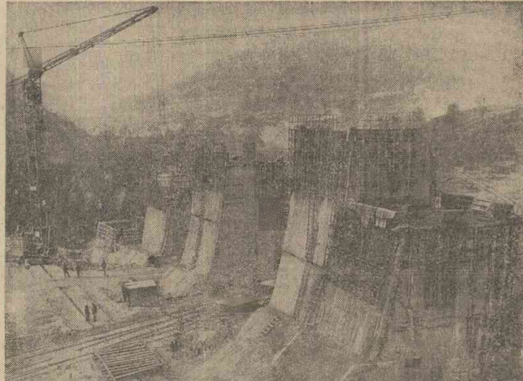
În Valea Doftanei continuă lucrările de betonare a barajului Paltinu. Aici, în spatele a 300 000 mc de beton va fi acumulat un volum de 56 milioane mc de apă, servind pentru asigurarea nevoilor de apă potabilă și industrială în zona orașului Ploiești. Foto: NICU, VASILE
