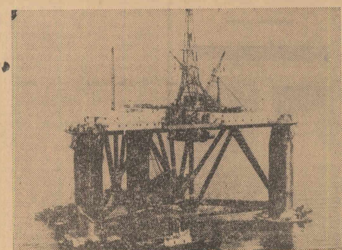
Forajul submarin, ale cărui principii sînt aproape identice cu cele aplicate la cel terestru, cu deosebire că se efectuează de pe o platformă, un fel de insulă artificială plasată în mare, capătul în ultima vreme o mai mare extindere. Recent, Șantierul naval din Hiroshima a realizat cea mai mare platformă submarină pentru exploatarea petrolului — fotografia noastră — pe care vor putea lucra 60 de persoane și vor ateriza elicoptere
