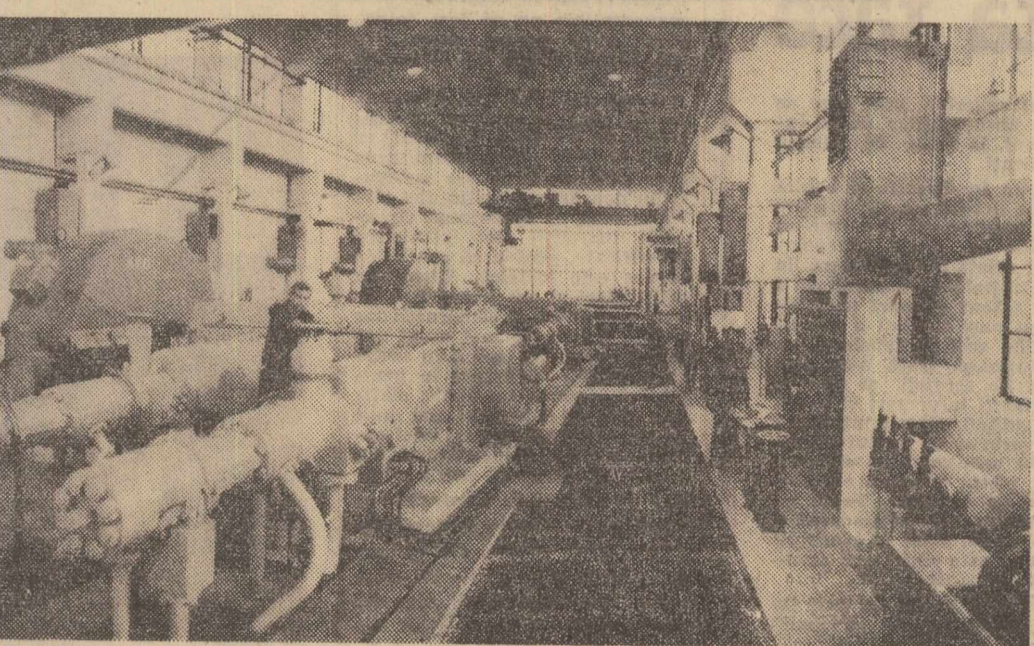
Combinatul chimic de la Tg. Mureș este una dintre cele mai moderne unități ale industriei chimice românești. Cliseul nostru vă prezintă sala compresorilor sinteză, executată în cadrul etapei a II-a de extindere a combinatului.
