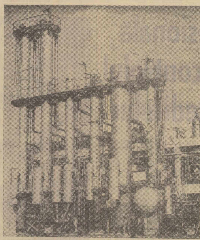
La Uzina de fibre sintetice din Iași, lucrările de construcții-montaj se află într-un stadiu avansat față de grafice. Aceasta va da posibilitatea începerii probelor tehnologice încă în cursul acestui an. Concomitent pe acest șantier au fost atacate la secția filare și depozitul fierului, lucrările etapei a II-a în cadrul căreia se vor produce 3000 tone fire textile din poliester. În clădire: Una din instalațiile de distilare a uzei.
