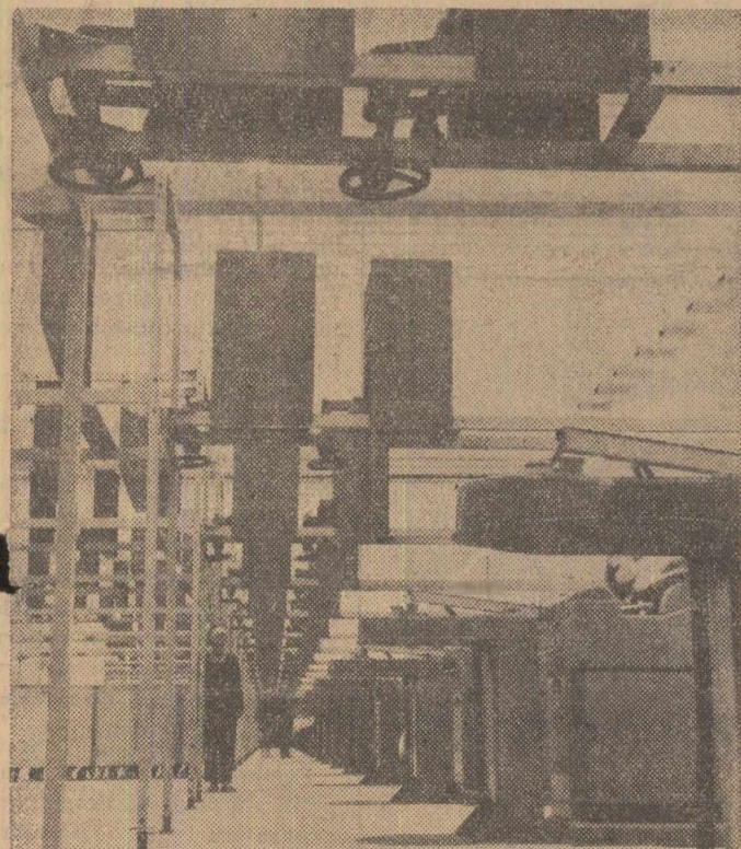
Devansarea cu circa 6 luni față de grafic, a lucrărilor de investiții pe șantierul Uzinei de fibre sintetice TEROM, din Iași face posibilă începerea probelor tehnologice încă în cursul acestui an. Pînă în prezent s-a terminat rodajul la parcul de rezervoare și stația de pompe, urmînd ca și alte secții să intre în probe. În clișeu: vedere din secția etirare a uzinei
