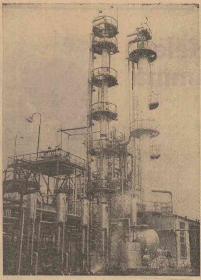
La instalația de fabricare a fenolului și acetonei, din cadrul Combinatului de cauciuc sintetic și produse petrochimice de pe Valea Trotușului, au fost executate ample lucrări de dezvoltare a capacităților de producție și de îmbunătățire a procesului tehnologic.
