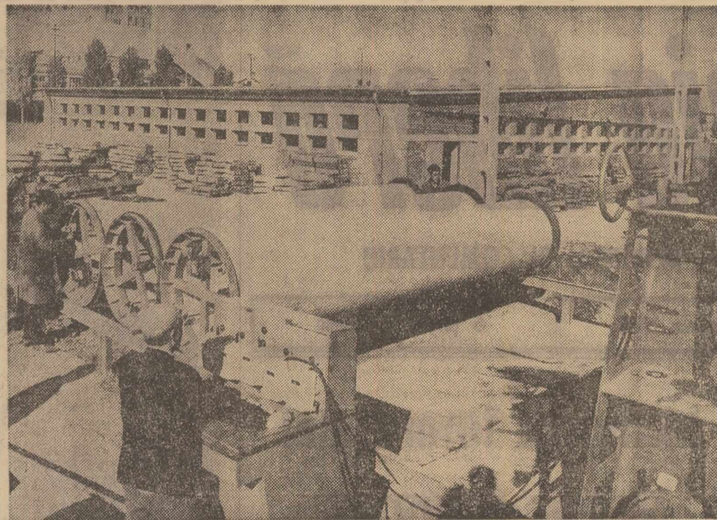
De curînd, s-a pus la punct o invenție românească — „instalația de aplicare a stratului de protecție la tuburi din beton precomprimat prin vibrataminare”, realizată în cadrul măsurilor de organizare științifică a producției pe acest an în întreprinderea de prefabricate „Progresul” din București. În clișeu nostru reproducem această instalație
