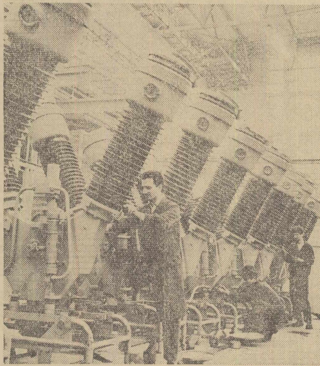
Uzina „Electroputere” Craiova și-a extins capacitatea de producție prin construirea, recentă, a unei noi fabrici de aparatură electrică. În clișeu: montarea interupătoarelor de 110 k.W produse în această fabrică, destinate stațiilor de înaltă tensiune
