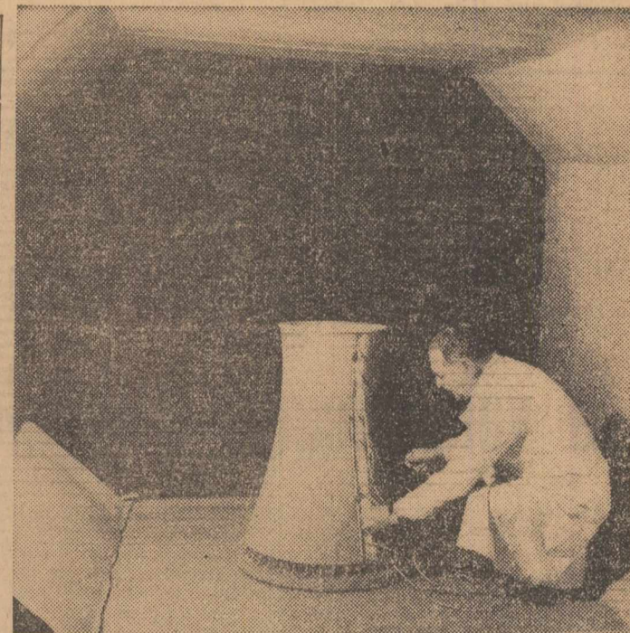
Cu ajutorul modernei și complexe aparatură ce le stă la dispoziție, cercetătorii Institutului de mecanică a fluidelor studiază și o serie de probleme cu aplicare directă în practică. Fotografia noastră vă înfățișează tocmai o astfel de operațiune în cadrul căreia, pe macheta unui tur de răcire de la Centrala termoelectrică Rovinari, se urmărește determinarea sarcinilor aerodinamice provenite din acțiunea vînturilor
