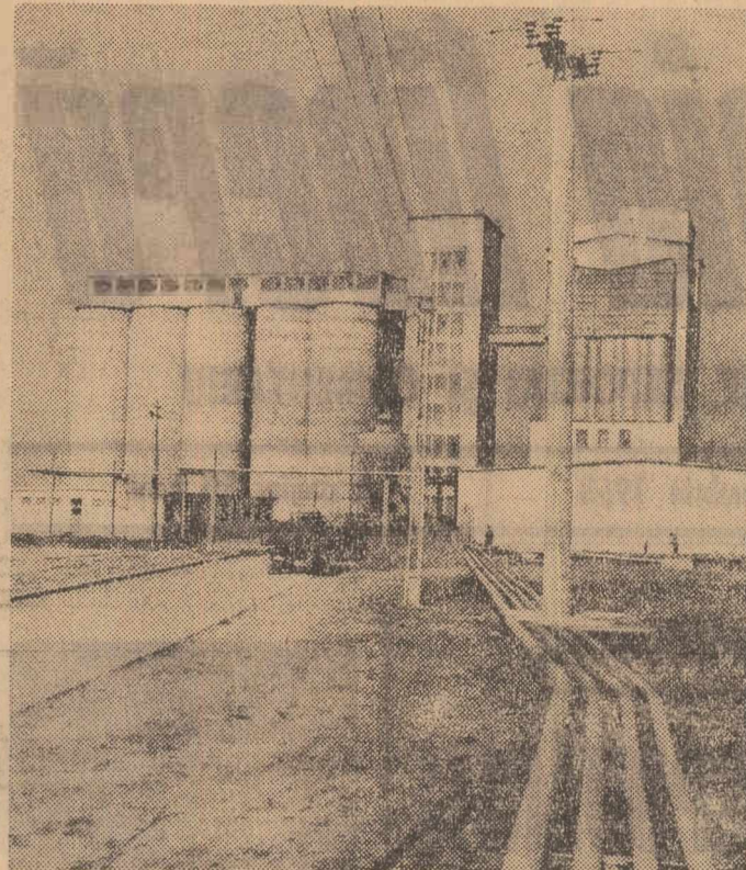
La întreprinderea agricolă de stat Peris, județul Ilfov, a intrat în producție în cursul acestui an o fabrică de nutrețuri combinate. În clișeu: Aspect exterior al noii unități industriale
