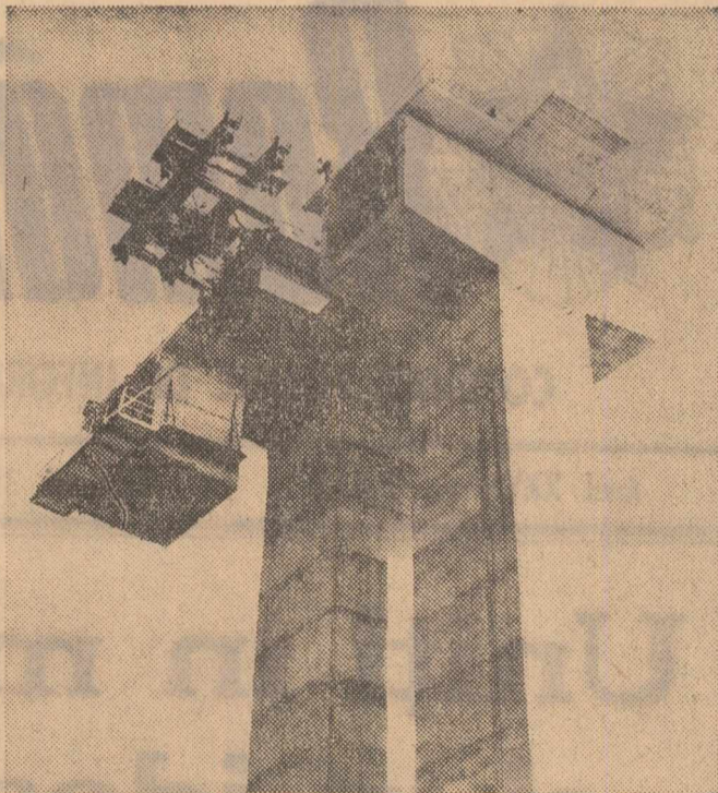
La viaductul Cătușa care va lega orașul Galați de Combinatul siderurgic, a început recent montarea primelor tronsoane prefabricate, cu dispozitive speciale proiectate și executate în țară, pentru montări de poduri în consolă
