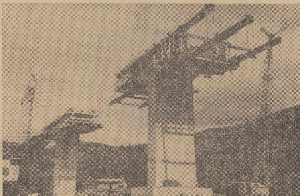
Cu sporită eficiență, activitatea cotidiană a constructorilor din cadrul șantierului I.C.P.F. 73 Orșova, se materializează în noi edificii destinate facilitării circulației rapide. Deasupra apelor Cernei se construiește un nou viaduct
