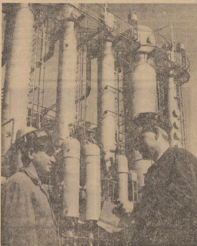
Pe șantierul Uzinei de fibre sintetice din Iași se lucrează intens la montarea instalațiilor. Noua uzină va intra în probă tehnologică la sfîrșitul trimestrului IV al anului curent. Cînd vor intra în funcțiune toate agregatele, uzina va avea o capacitate de 10.000 tone fibre pe an. În clișeu: Aspect de pe șantier
