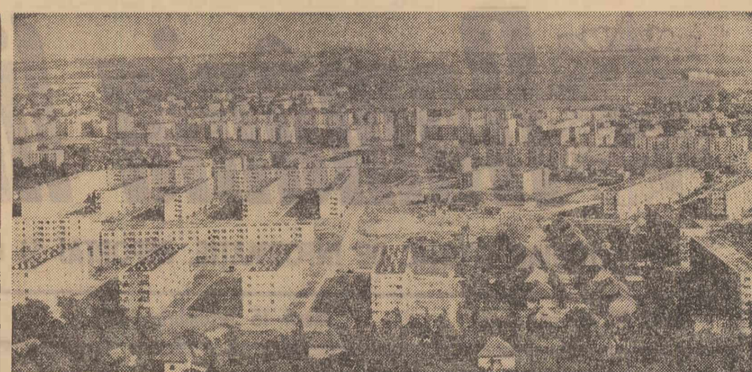
Cartierul Săsar din Baia Mare
