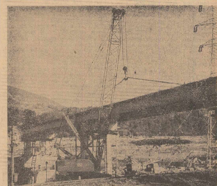
La podul ce se construiește peste Jiu — în drumul către mina Paroșeni — se lucrează în prezent la montarea uriașelor grinzi de beton armat.
