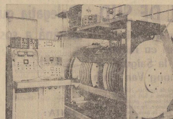
In atelierele centrale ale Institutului de fizică atomică s-a construit un electromagnet cu câmp magnetic, în greutate de 12 tone, folosit pentru lucrări de radiospectroscopie, în special pentru studii de polarizare dinamică a nucleelor.
