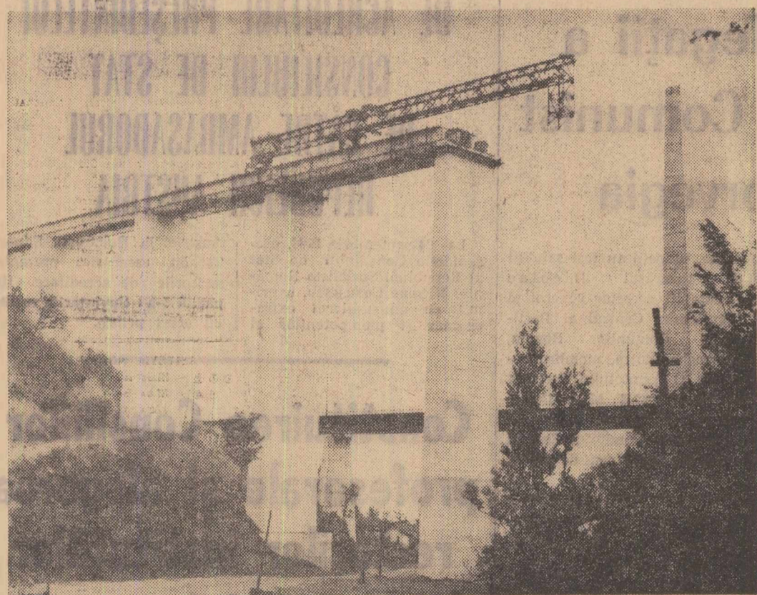
O soluție pentru montarea grinzilor din beton la poziții înalte și inaccesibile macaralelor sau altor mecanisme. Aspect de la viaductul Slătinești-Mare în construcție pe porțiunea Tr. Severin-Orșova Foto: FLORIN ȘTEFĂNESCU
