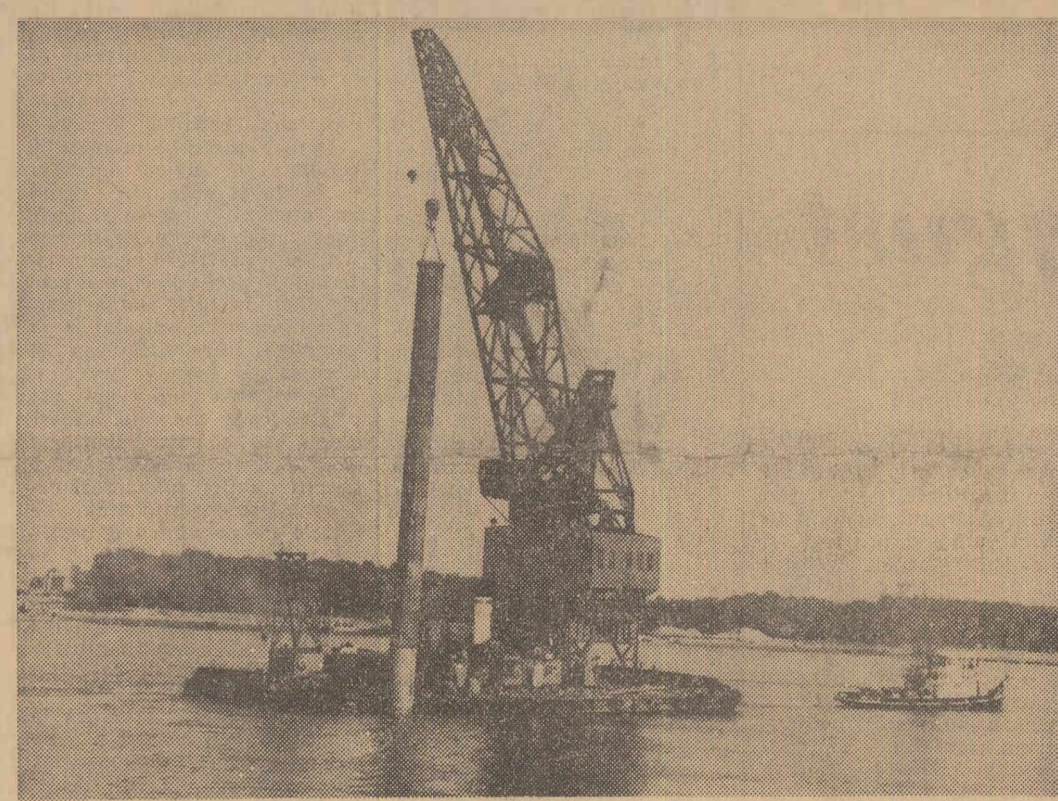
Construcția podului peste Dunăre — între Giurgeni și Vadul Oii — impune amenajarea unei insule artificiale care să permită lucrul la pilele „albă” în clisău: Transportul coloanelor de susținere ale platformei autoridicătoare care va constitui „insula” din mijlocul fluviului pentru lucrările în zona Giurgeni
