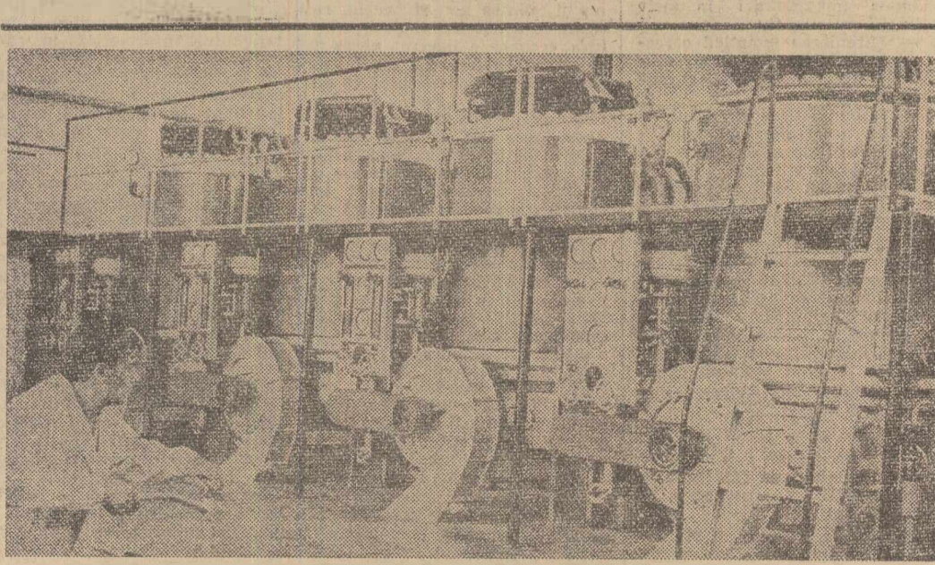
Centrala termică a Institutului de fizică atomică din București-Măgurele a fost echipată cu cazane de tip GAMA de mare randament, proiectate în institut. În prezent, acest tip de cazane se află în producție de serie la Uzina „16 Februarie” Cluj. Fiecare cazan are un debit de 2.000.000 kilocalorii pe oră și un randament de 92 la sută
