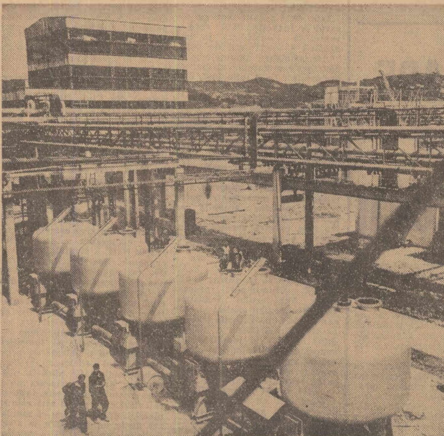
Vedere parțială a Combinatului chimic din Rm. Vâlcea Foto: AGERPRES
