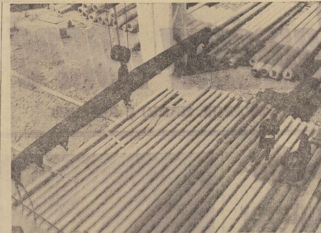
Fabrica „Titan” este singura unitate din ţară profilată în fabricarea stîlpilor de beton pentru linii electrice de înaltă tensiune. Secţia de fabricare a stîlpilor centrifugaţi din beton precomprimat asigură produselor o calitate superioară. În clădire: aspect din depozitul de produse finite al fabricii.
