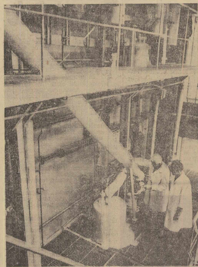
La Uzina chimică Duceşti, s-a pus la punct un nou procedeu de fabricare a polietilenei de joasă presiune, graţie a unui echipament deosebit. De asemenea, se experimentează un nou procedeu de fabricare a glicerinei sintetice. În clădire: seful colectivului de cercetări Ing. Emil Alexandrescu şi Fl. Bărbăneanu urmînd procesele tehnologice
