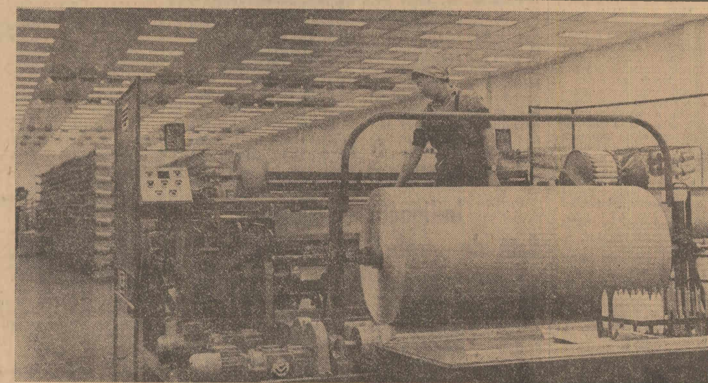
În cadrul uzinei din Săvinești, la secția poliamid a noii fabrici Relon III a început de curînd montajul mașinilor de polimerizare și filare care vor produce anual 100 de tone fire textile. Tehnologia de fabricație este stabilită pe baza experimentărilor efectuate la Relon I și II. În clișeu: Aspect de la fesoția fabricii Relon II Foto: MIHAI POPESCU
