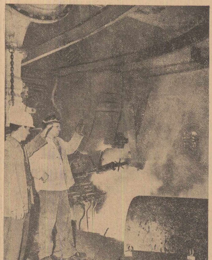
La Combinatul siderurgic din Galați s-a montat prima virolă a corpului metalic de la cel de-al doilea furnal de 1700 mc, aflat în construcție. Experiența acumulată la primul furnal a făcut ca ciclul de realizare a construcției — până la stadiul de montaj — să fie considerabil scurtat. Concomitent, se acordă o deosebită atenție desfășurării procesului de producție la capacitățile existente. În clădirea Ingerului Ion Vasile și prim-topitorul Ion Blaj, urmând descărcarea unei șarje de fontă la primul furnal de 1700 mc
