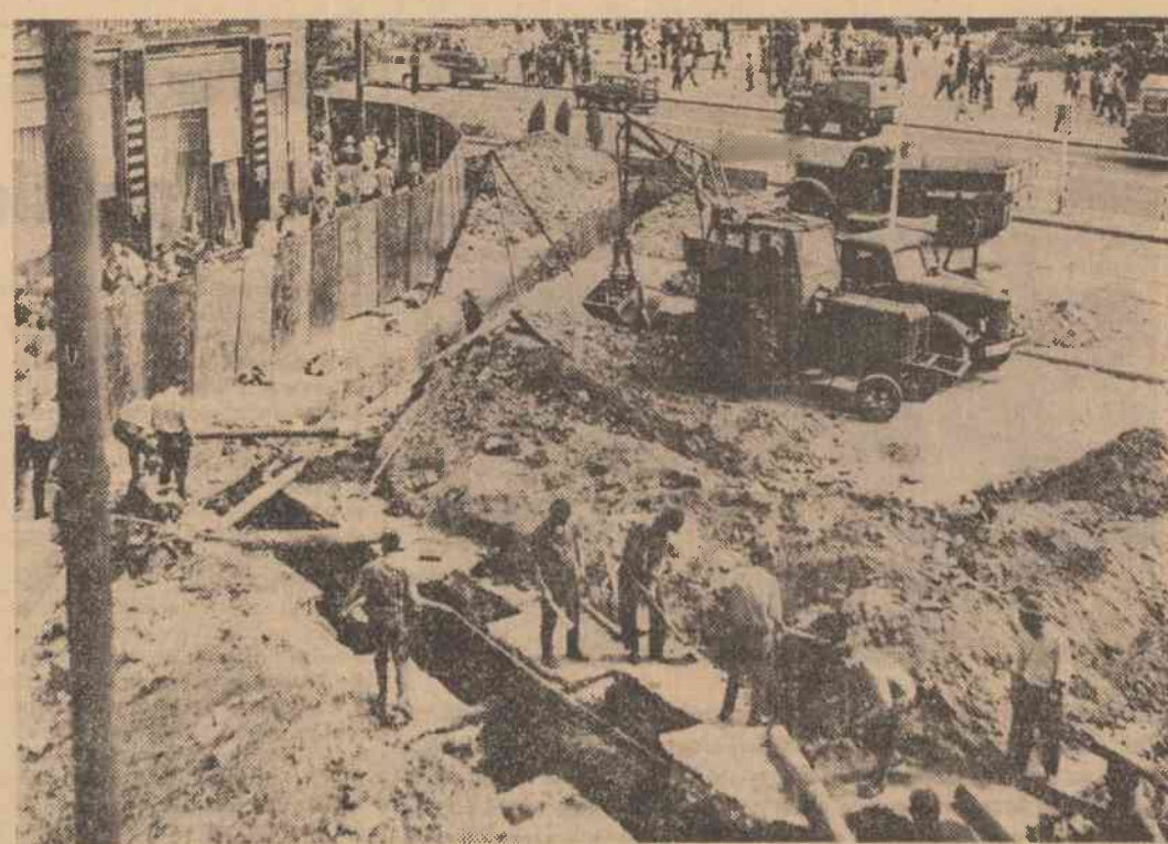
În Capitală în Piața 1848 se construiește primul pasaj subteran pietonal, care va traversa bulevardul 1848. În clipă: Aspect de pe șantierul viitorului pasaj
