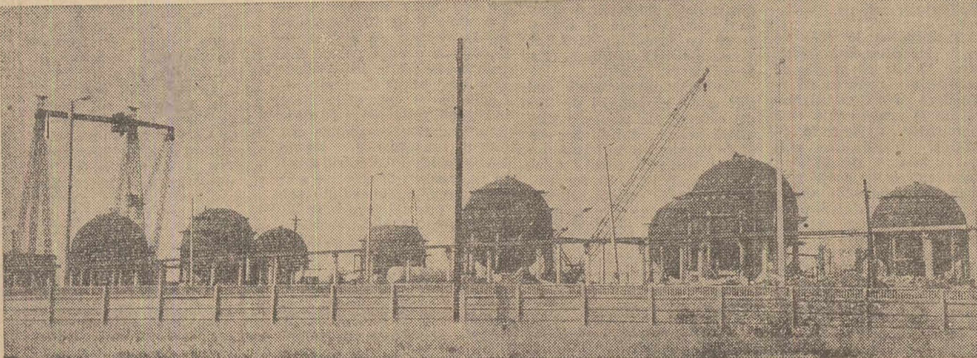
Rezervoare sferice la Combinatul petrochimic Pitești
