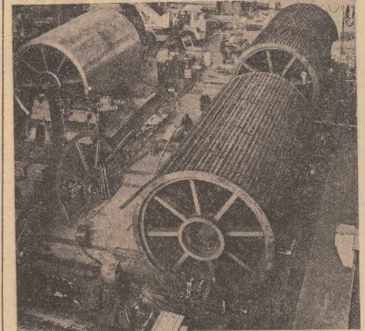
Începînd din acest an firma suedeză Karlsdats Mekaniska Werkstad a început producerea în serie a unor filtre gigantice, necesare hidrocentralelor din ce în ce mai mari care se construiesc în diferite părți ale lumii. Filtul din imagine are un diametru de 4 metri și o lungime de 14 metri și, pentru a se putea transporta mai ușor, se confecționează din două bucăți. Capacitatea nominală de filtrare a agregatului este de 920 tone în 24 de ore, dar, după cum informează producătorii, în curînd vor proiecta filtre și mai mari, de peste 1 000 tone.
