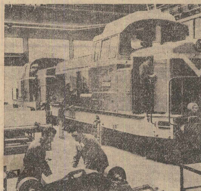
Construcții de locomotive de la Uzinele „23 August” au realizat recent un nou tip. Este vorba de locomotiva Diesel hidrolică 1 200 CP, care se fabrică în serie. În cliseu: Finisarea locomotivelor în hala de montaj general
