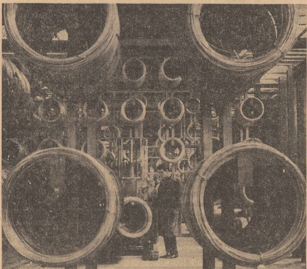
La Uzina de sîrmă din Buzău a intrat în exploatare sectorul de fabricat sîrmă pentru electrozi. Utilajele — amplasate în flux tehnologic — dau posibilitatea ca procesul de fabricație să fie direcționat de un număr restrîns de lucrători, alimentarea, reglarea, traficul și debitația sîrmei efectuîndu-se automat. Tot în cadrul uzinei a început montajul a trei linii tehnologice, dotate cu instalații și utilaje automate Foto: NICU VASILE
