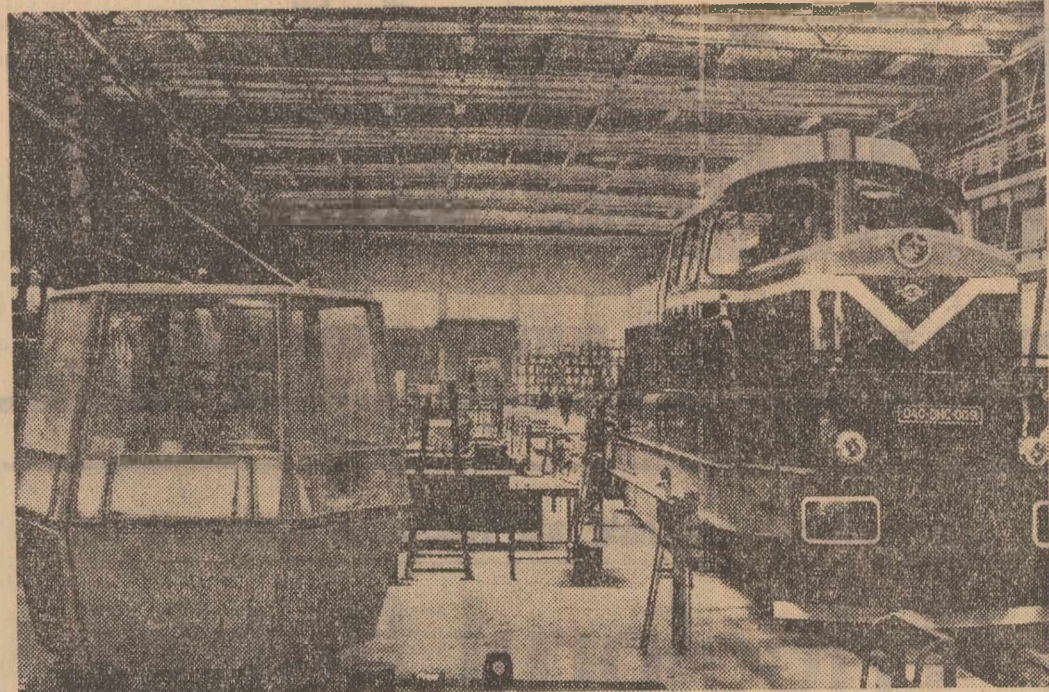
Uzinele „23 August“ din Capitala. Printre produsele bine apreciate, care se fabrică aici se numără și locomotivele Diesel hidraulice de 350 CP, 750 CP și 1250 CP. În clădirea a nouă locomotivă Diesel hidraulică de 1250 CP este pregătită pentru a ieși pe porțile uzinei.
