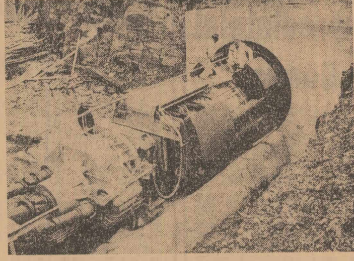
O gigantică mașină de forat, lungă de 31 metri și avînd o greutate de 115 tone, a fost pusă recent în funcțiune la lucrările de construcție a unui tunel de 7,5 km care va lega rezervorul de apă Oker cu cel din valea Grane aflat, în construcție, lângă Goslar Har, în nordul R.F. Germaniei. Tunelul, care va avea un diametru de 3,15 metri, va fi terminat în doi ani. Viteza de penetrație a acestei mașini este de 4 metri pe oră.
