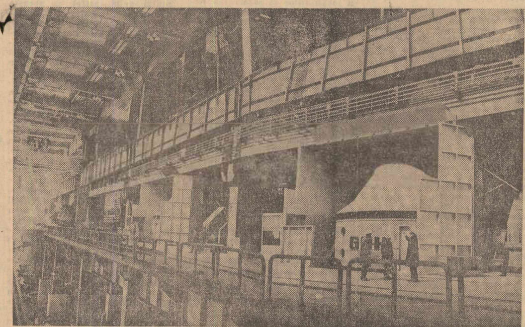
Platforma convertizoarelor de la noua oțelărie a Combinatului siderurgic de la Galați. Ieri înaintea ivirii zorilor aici s-a elaborat șarja inaugurală. Foto: NICU VASILE
