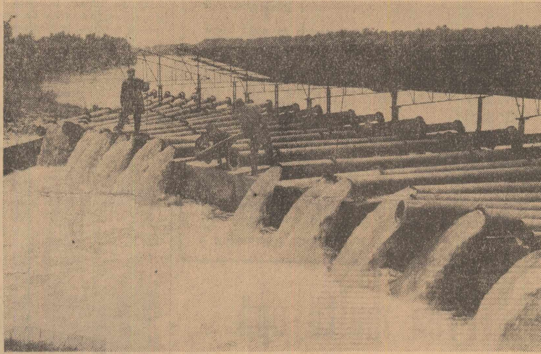
Stația de pompare a sistemului de hidroameliorații Drăgănești, județul Olt, irigă peste 500 ha culturi de cimp și peste 700 ha de orez. Foto: AGERPRES
