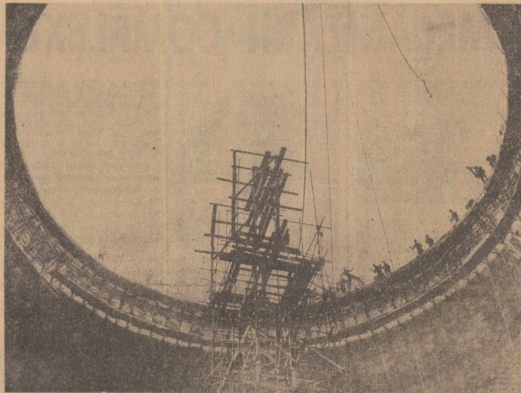
Pas cu pas, către cota finală... În cliseu: turnul de răcire a apei în construcție pe șantierul Rafinării Pitești.
