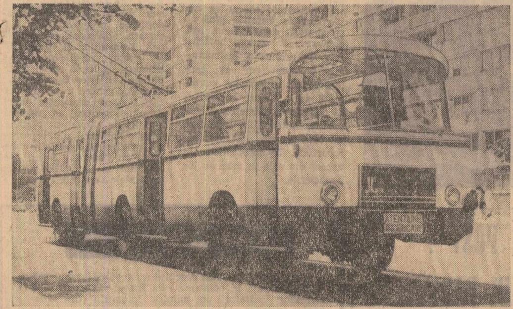
Pe străzile Capitalei circula de câteva zile două troleibuze articulate, realizate de uzina „Autobuzul” în colaborare cu Fabrica de mașini electrice și „Electroaparat”. Noile troleibuze au o capacitate de 190 pasageri, pot dezlota o viteză de 55 km. pe oră, prezentînd totodată caracteristici îmbunătățite față de tipurile actuale. În clipă: Unul din cele două troleibuze
