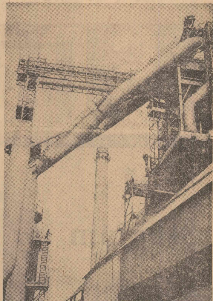
O imagine impresionantă, devenită familiară constructorilor Com-binatului siderurgic de la Galați: furnalul de 1700 m.c.
