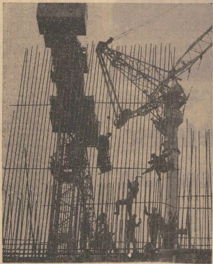
Pe șantierul mariei cetăți a luminii de pe Dunăre, la Porțile de Fier, lucrările continuă să se desfășoare din plin. În clipă : Aspect de la betonarea capului intermediar al ecluzei și capului aval pentru deschiderea frontului de lucru în vederea montării pieselor metalice din echipamentul hidroenergetic
