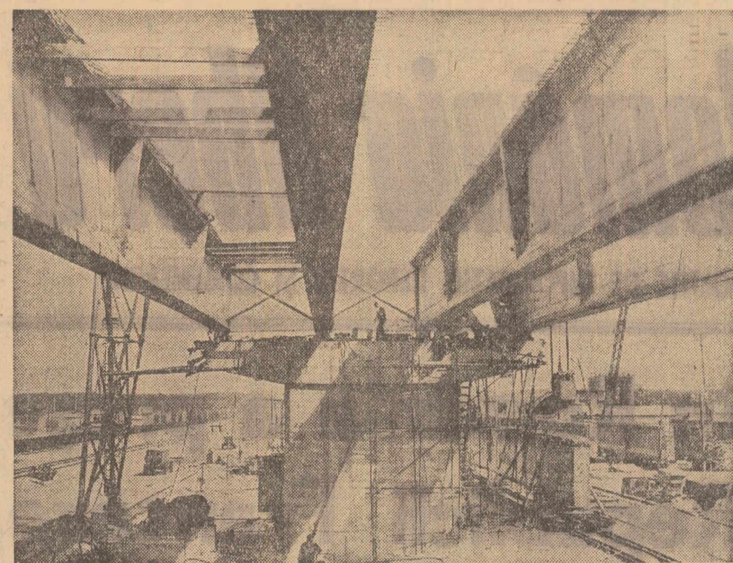
Lucrările de construcție la podul rutier peste Dunăre sînt în plină desfășurare. Imaginea pe care o prezentăm astăzi redă un aspect din zona de viaduct de la Giurgiu. Primele grinzi de beton armat precomprimat au fost ridicate pe piloni. Foto: NICU VASILE
