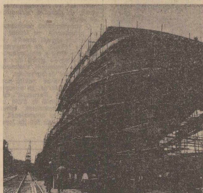
La Uzina mecanică Turnu Severin a început, pentru prima dată, construcția unor cîrcori de 2.200 tone cu magazie frigorifică, dotate cu aparatură și instalații moderne. În clipă: Un aspect de la sala de montaj și lansare a cîrcorilor. Foto: AGERPRES
