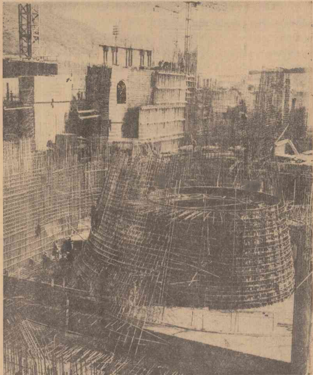
Lucrări la ecluza de la Porțile de Fier
