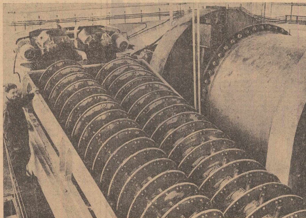
Clasorul spiral a tulburării de minereu de la întreprinderea Fundul Moldovei, județul Suceava.
