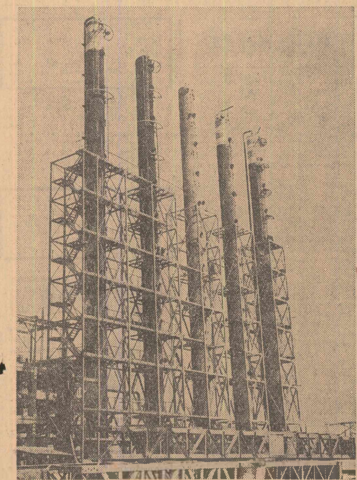
Coloanele de separare a xilenilor din cadrul complexului de reformare catalitică de la rafinăria din Pitești
