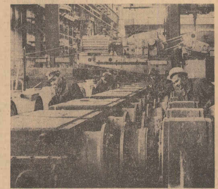
În clipă: Un grup de muncitori montează căile cu role din fața și din spatele caiei principale a laminorului bluming de 1300 mm. Foto: MIHAI POPESCU
