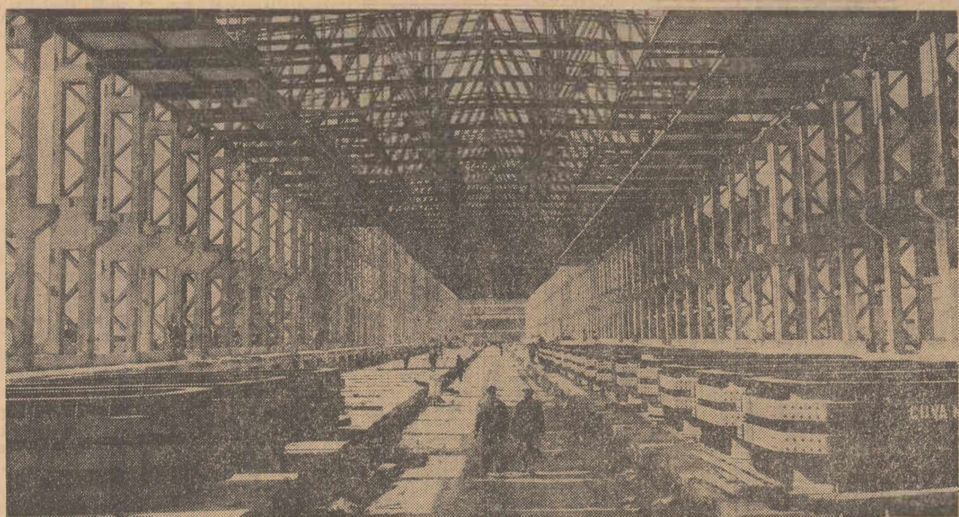
O imagine din aceste zile a stadiului lucrărilor de construcții și montaj de la etapa a III-a de dezvoltare a Uzinei de aluminiu din Slatina
