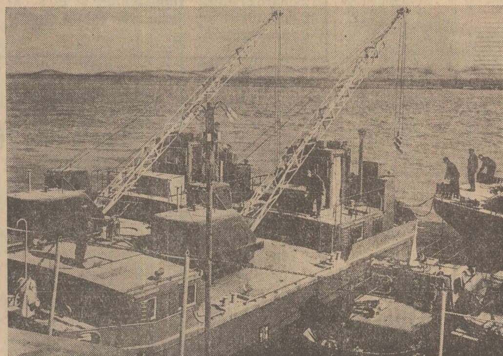
Fotografia noastră vă prezintă un nou produs al Șantierului naval din Brăila, vasul pentru manipularea sarcinilor ușoare. Dotat cu un excavator de 0,3 mc și echipament de ridicare acest nou tip de vas efectuează lucrări de transbordare, încărcare și descărcare, fiind deosebit de util în condițiile de navigație ale Deltei Dunării.
