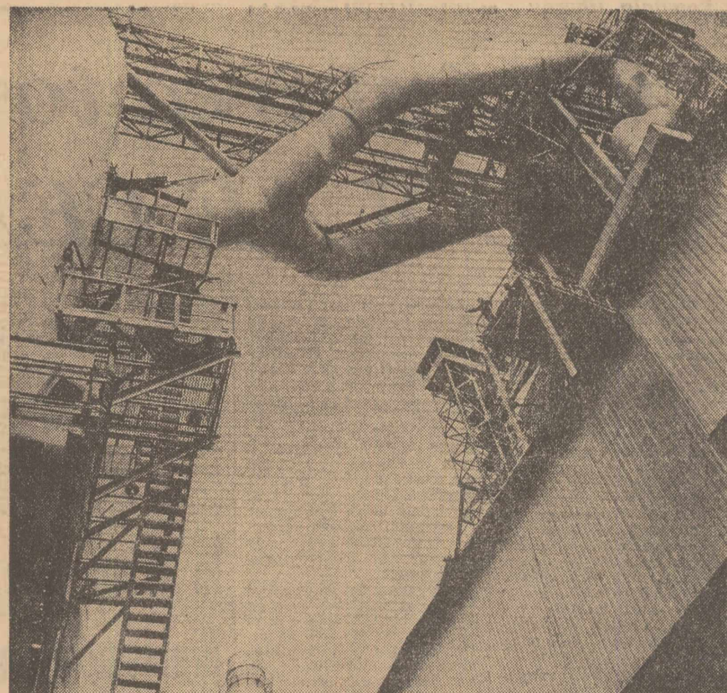
Colosul de 1 700 m.c. în așteptarea evenimentului: prima șarjă de fontă.
