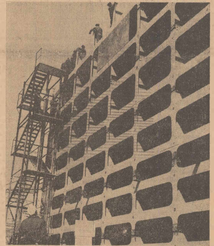
Asemeni unui imens fagure de oțel înalt de 34 m, porțile buscate din aval ale ecluzei se făuresc de către oameni. Este o replică contemporană a Porților de Fier
