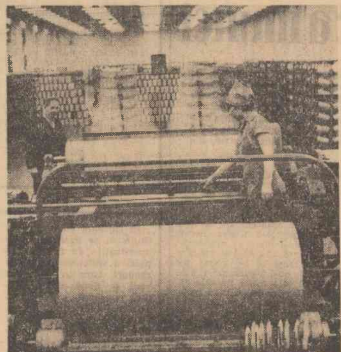
Interior industrial modern la Relon II — Uzina de fibre și fire sintetice-Săvești. Fiecare din războaiele semiautomate instalate în atelierul de jesut cord produce, pe oră, 48 metri țesătură pentru pinzele de anvelope
