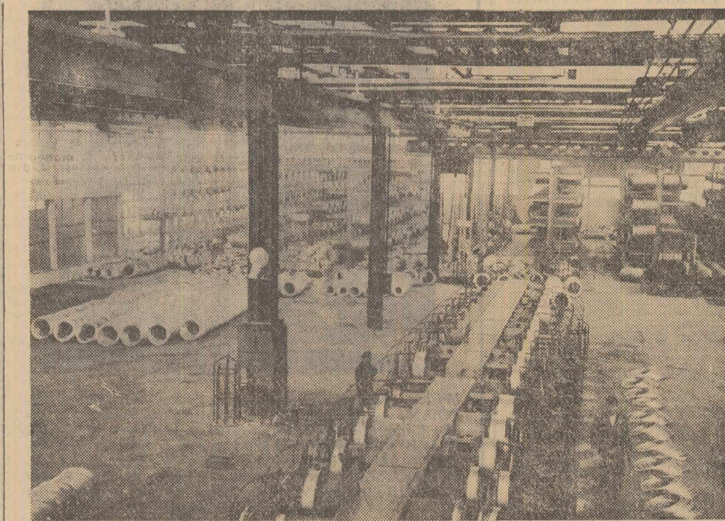
Printre cele mai tinere obiective industriale din Buzău se numără și Uzina de sîrmă. Noua unitate, intrată în funcțiune în 1967, se dezvoltă în continuare prin intrarea în funcțiune a unor moderne capacități de producție. În clișeu: linia de zincat a sîrmei laminată.
