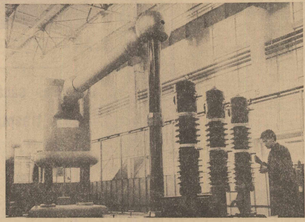
La uzinele Electroputere din Craiova a intrat în funcțiune o instalație complexă — pe care v-o prezentăm în imagine, destinată verificării aparatelor electrice. Înalta tehnicitate a aparatelor — oscilografe, oscilometre, pupitre de comandă programate, — permite un control complet și riguros al produselor destinate a funcționa la tensiuni până la 500.000 de volți.
