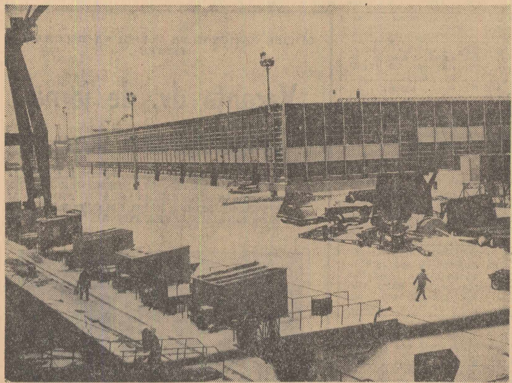
În curînd, la şantierul naval din Galaţi va intra în funcţiune o hală de armare care va grupa toate atelierele ce colaborează la armarea şi finisarea navelor. Lucrările se află acum în fază de finisaj. În imagine: aspect general exterior al halei de armare.
