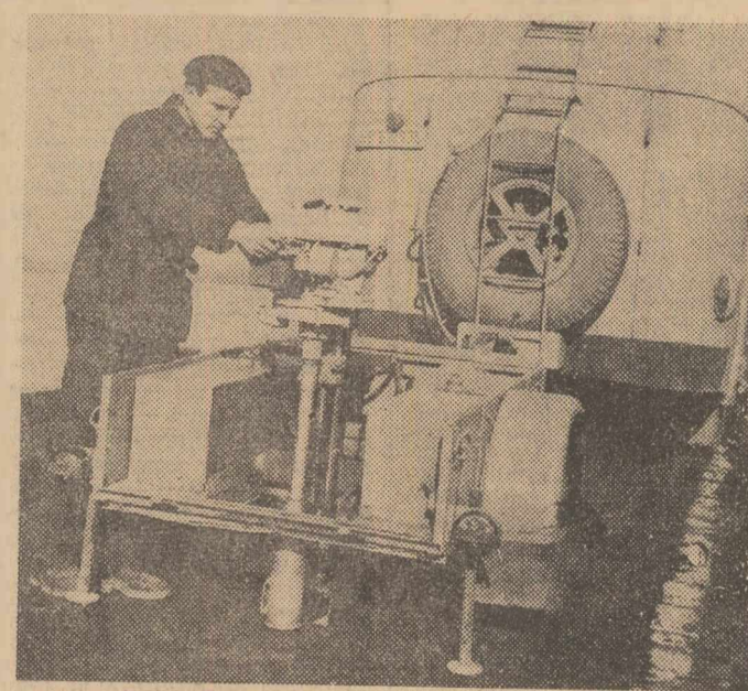
În vederea verificării calității execuției drumurilor, Institutul de cercetări în transporturi întreprinde — așa cum se vede în clișeu — încercări cu ajutorul unor utilaje adecvate
